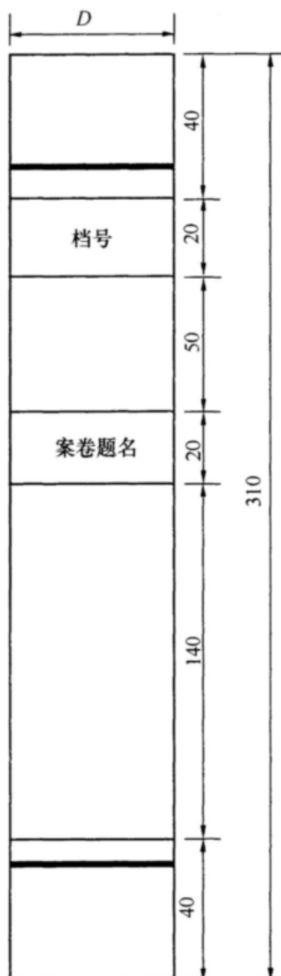
图 F 案卷脊背式样
