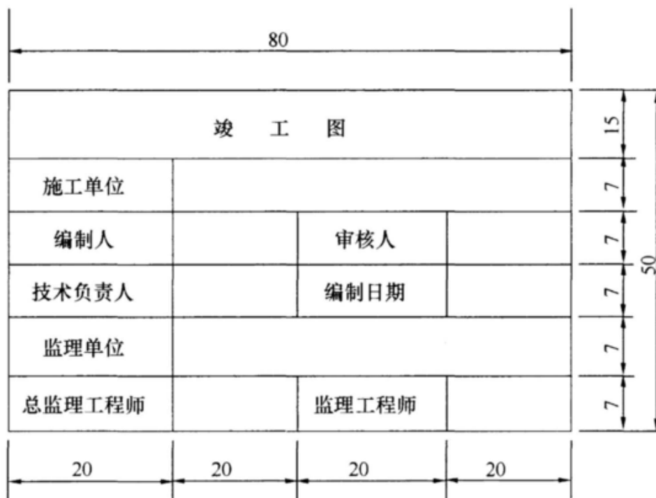
图 4.2.8 竣工图章示例
